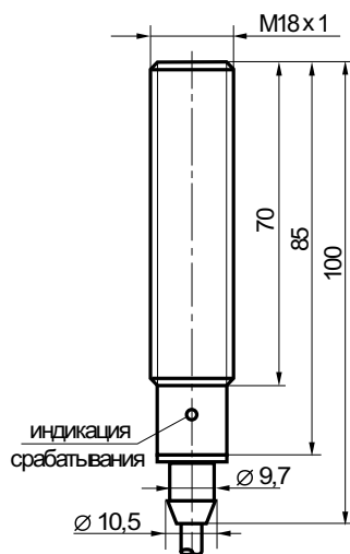
Габаритный чертеж.
