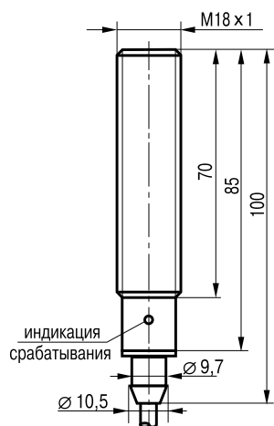
Габаритный чертеж.
