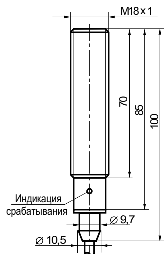
Габаритный чертеж
