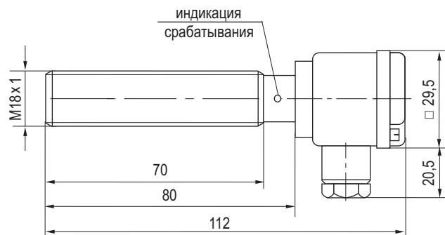
Габаритный чертеж
