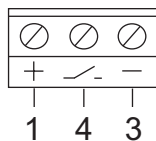
Маркировка клемм
