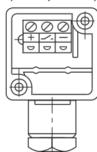
Маркировка клемм
