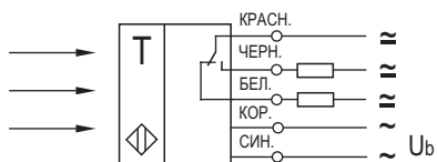
Схема подключения
