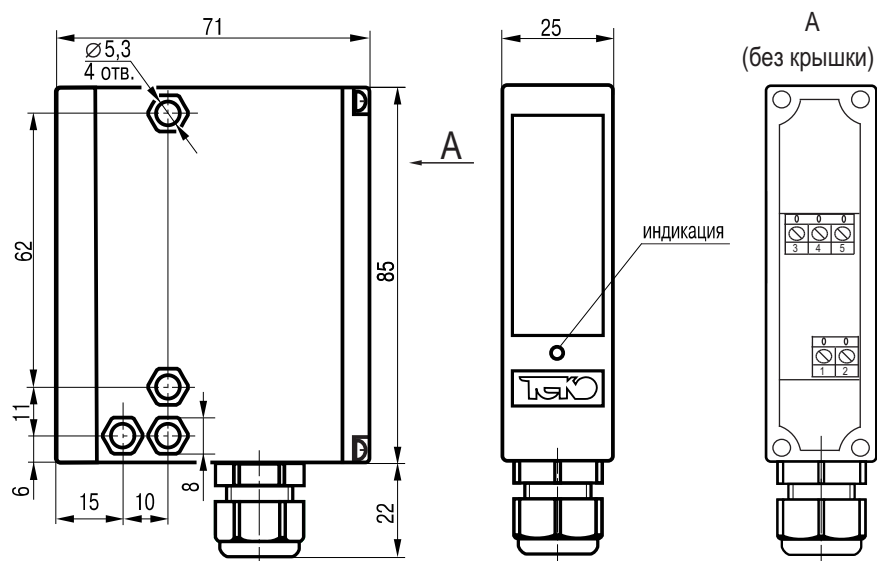
Габаритный чертеж
