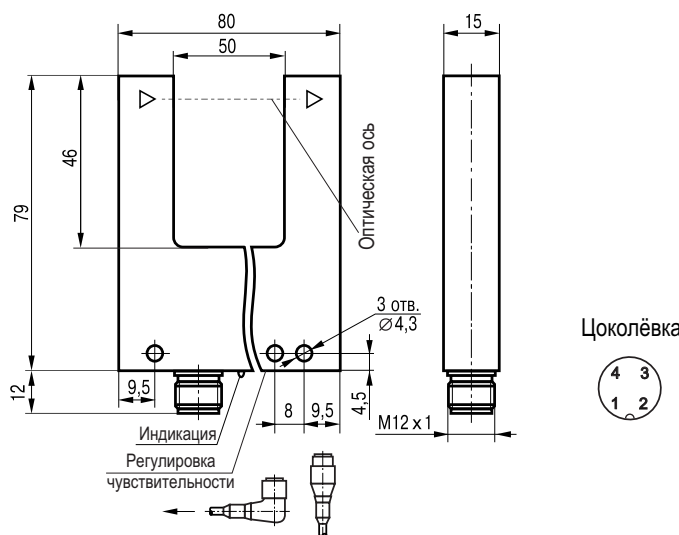
Габаритный чертеж
