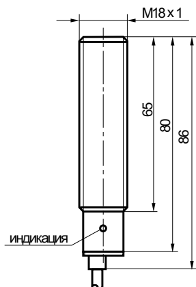
Габаритный чертеж.
