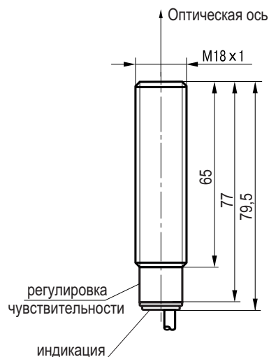
Габаритный чертеж.
