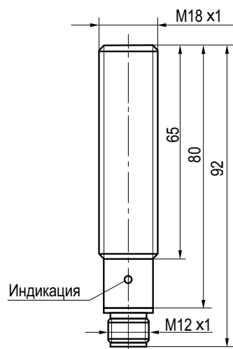
Габаритный чертеж.
