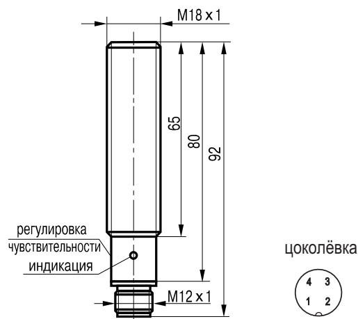
Габаритный чертеж.
