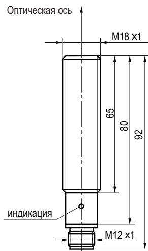
Габаритный чертеж.
