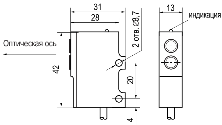
Габаритный чертеж.
