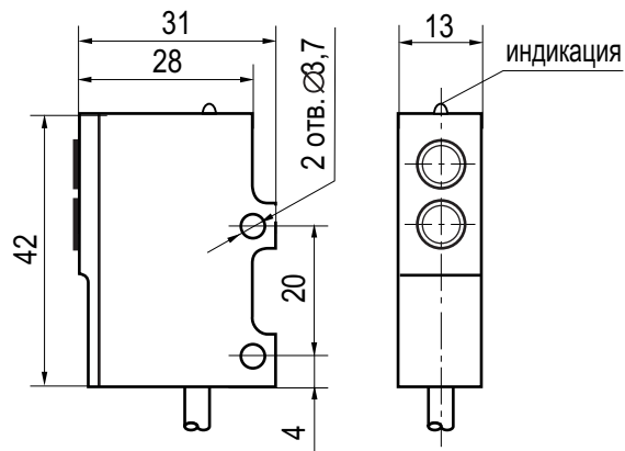
Габаритный чертеж
