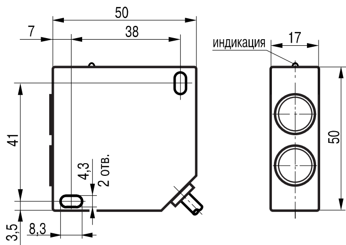
Габаритный чертеж
