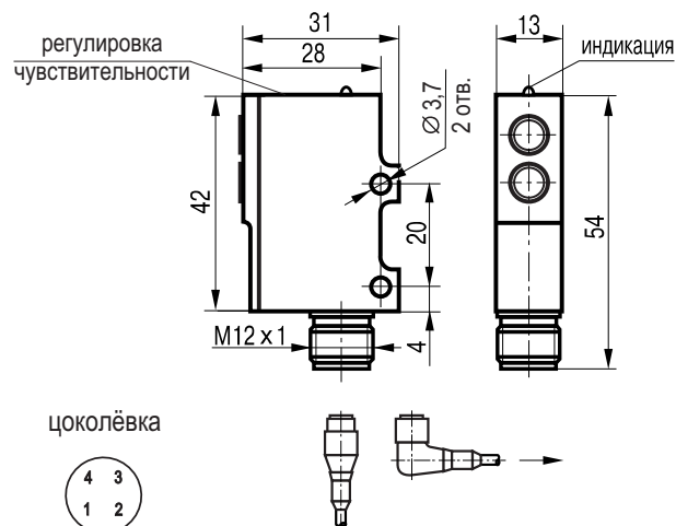
Габаритный чертеж
