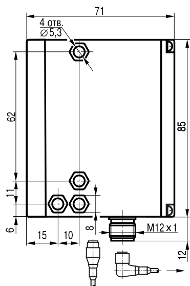
Габаритный чертеж
