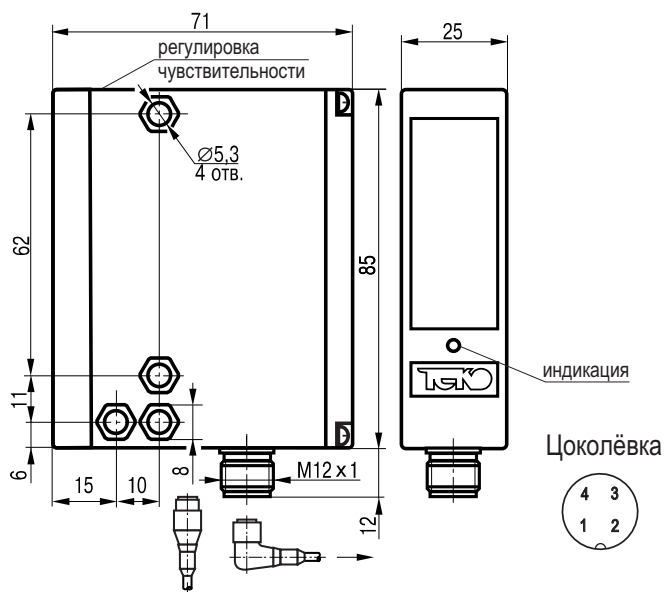
Габаритный чертеж.
