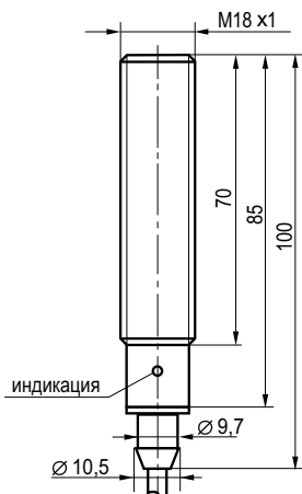
Габаритный чертеж
