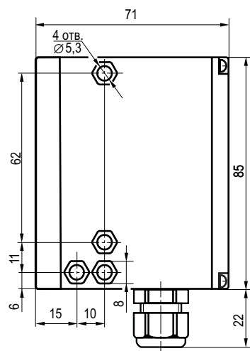
Габаритный чертеж
