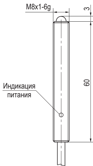
Габаритный чертеж
