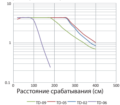
Рефлекторные с поляризацией (PSS/PSM-PM.../-E2)
