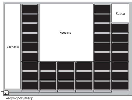
Рисунок 5. Общая схема подключения нагревательной пленки к терморегулятору в случае расположения установочных проводов непосредственно под напольным покрытием без дополнительной защиты от механических воздействий (вид снизу).
