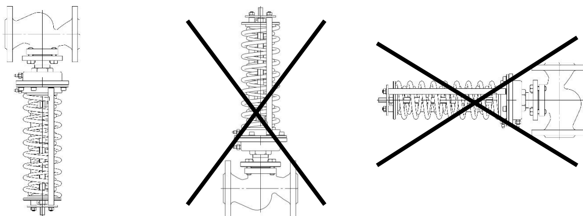
Рисунок А.4 - Монтажные положения регулятора на трубопроводе при температуре среды выше 120 °С (Прямолинейные участки до и после регулятора не требуются)
