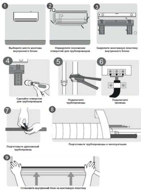
Рис.11 Краткое описание этапов монтажа внутреннего блока
