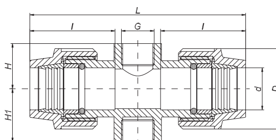
FEMALE TEE WITH PEG FITTING 90° T-STÜCK MIT INNENGEWINDE ABGANG UND ANSCHLUSS FÜR STANDROHRE Т-ОБРАЗНОЕ СОЕДИНЕНИЕ, РЕЗЬБА ОХВАТЫВАЮЩ., С КРЕПЛЕНИЕМ ДЛЯ СТОЙКИ
