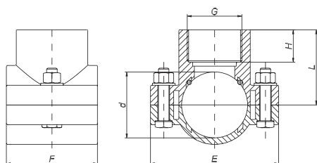
CLAMP SADDLE ANBOHRSCHELLE СЕДЛО ЗАЖИМНОЕ
