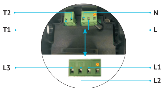
Рисунок 6 – Расположение клемм
