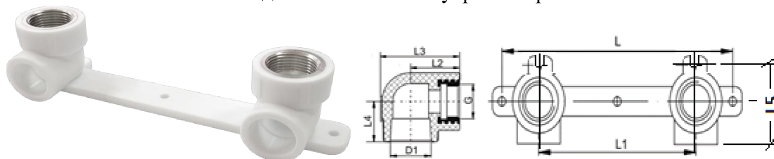
Рисунок 11. Настенный комплект для смесителя с внутренней резьбой.
