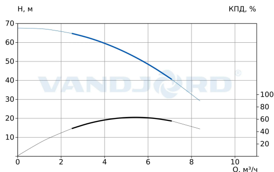
При заказе CRV 5-10A A-D-E-HQQE-A
