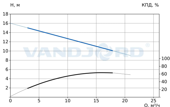
При заказе CRV 15-1B A-D-E-HQQE-E
