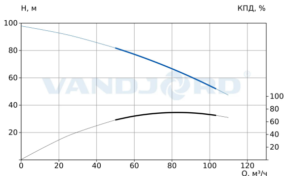
При заказе CRV 90-3B A-D-E-HQQE-E
