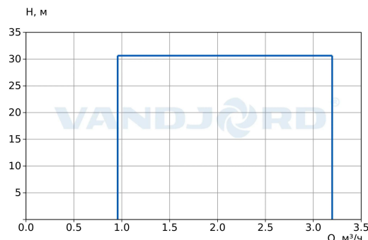
При заказе DMCS 3200-3 L-F-P-1-E
