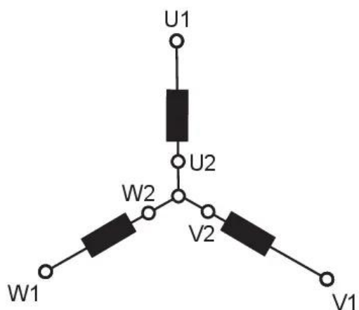
Соединение звездой
