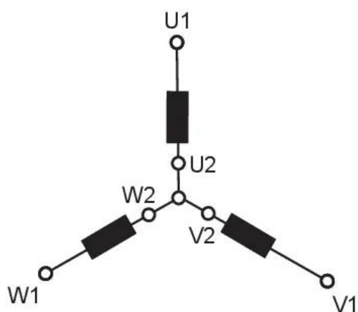
Соединение звездой
