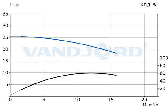
При заказе TPV 32-210-1.5/2 В-А-В-Е
