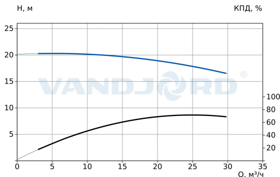
При заказе TPV 50-180-2.2/2 В-А-В-Е
