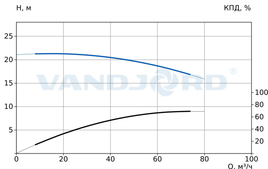
При заказе TPV 80-190-5.5/4 Q-A-B-E
