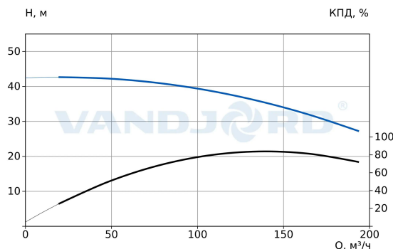
При заказе TPV 100-320-22/2 Q-A-B-E
