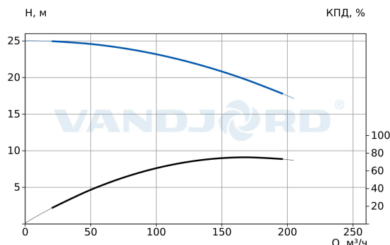
При заказе TPV 125-200-15/4 Q-A-B-E
