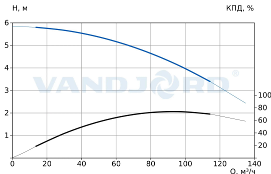
При заказе TPV 125-50-1.5/6 Q-A-B-E
