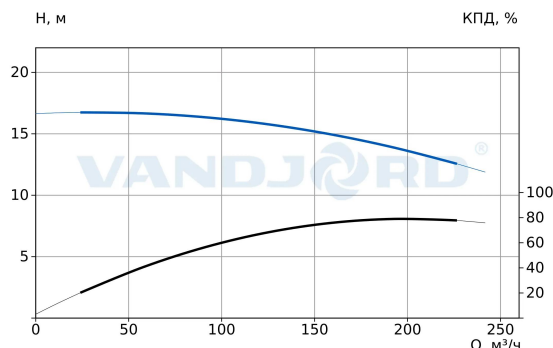
При заказе TPV 150-140-11/6 Q-A-B-E
