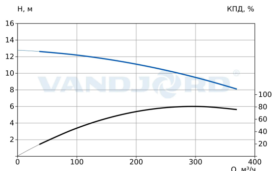
При заказе TPV 200-90-11/6 Q-A-BT-E
