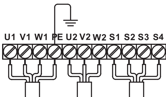
Подключение звезда/треугольник
