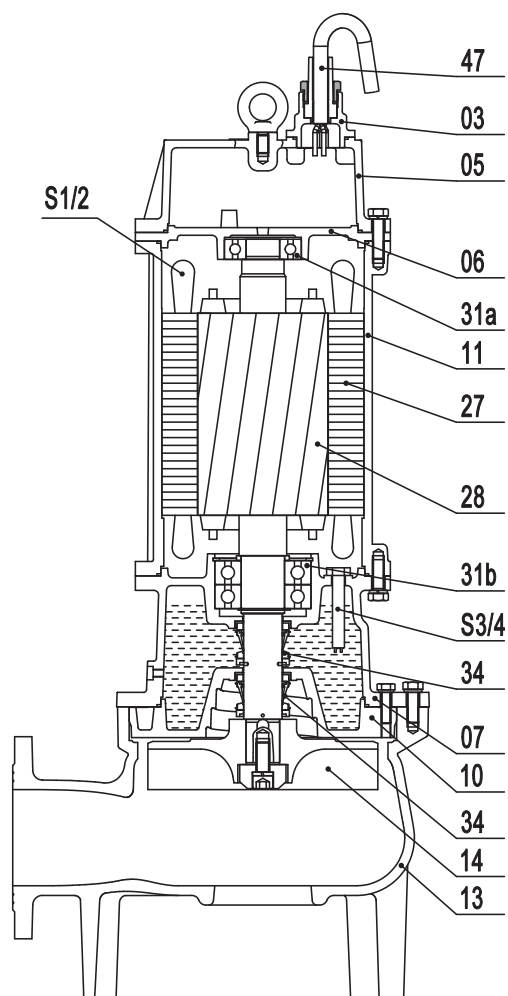
VSV 11,0 кВт
