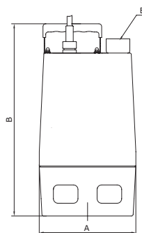
APV.40 (с охлаждающим кожухом)
