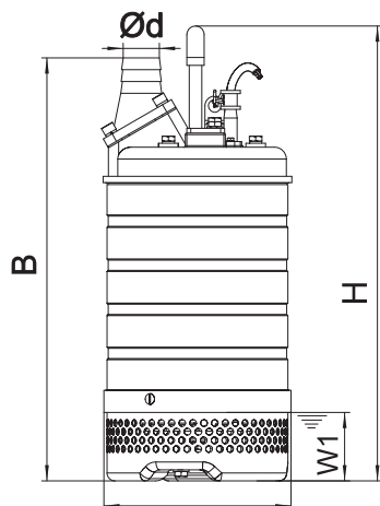
ØD 1,5–2,2 кВт
