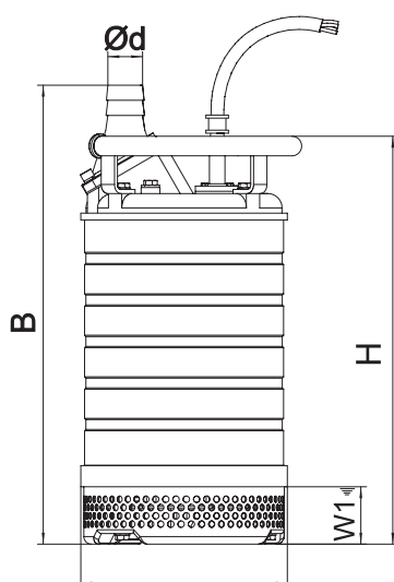
ØD 3,7–5,5 кВт
