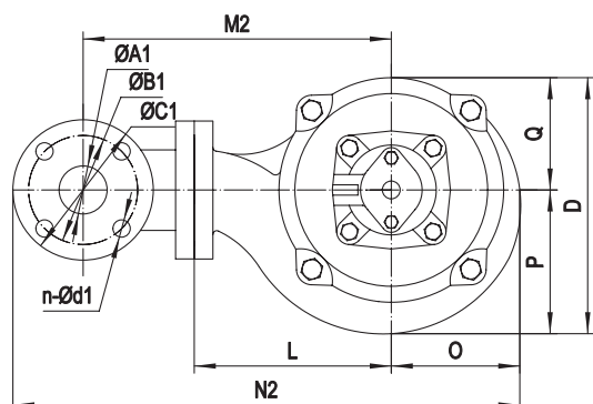
Размеры напорного патрубка насоса
