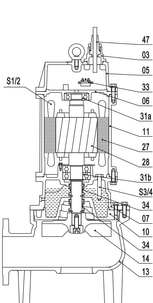
VSV 5,5–7,5 кВт
