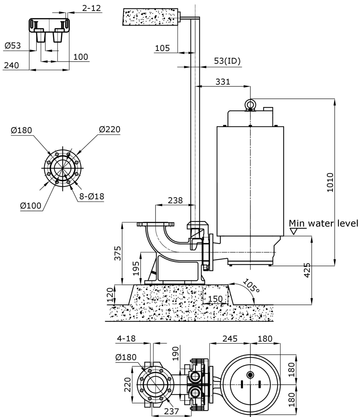
Габаритный чертеж VSE.100.185.2.C.192.N.5.1D.E
