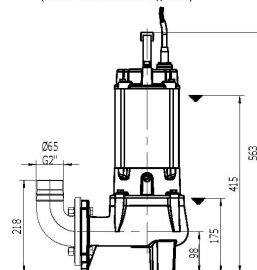
Переносная установка (колено заказывается отдельно)
