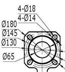
Фланец насоса PN 6/10
