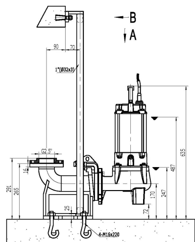
Установка на автоматической трубной муфте
