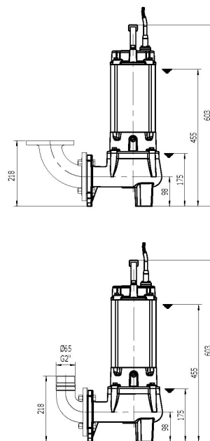
Переносная установка (колено заказывается отдельно)
