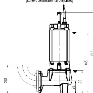
Переносная установка (колено заказывается отдельно)
