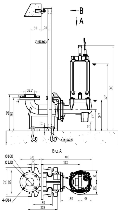
Установка на автоматической трубной муфте
