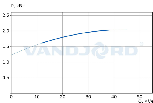
VSV - Канализационные насосы с вихревым рабочим колесом
