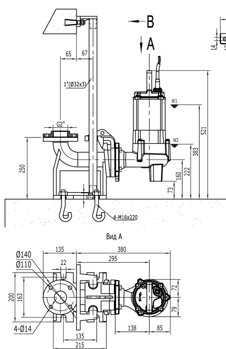
Установка на автоматической трубной муфте
